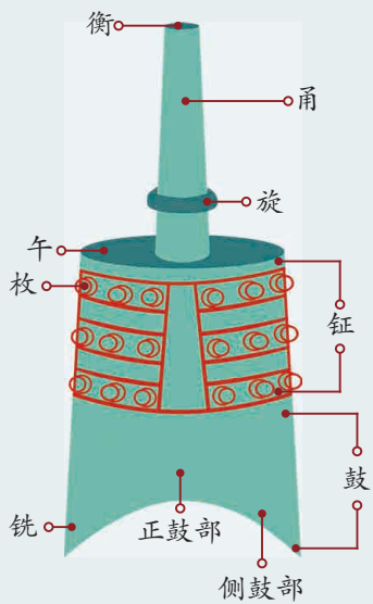
曾侯乙编钟构造
