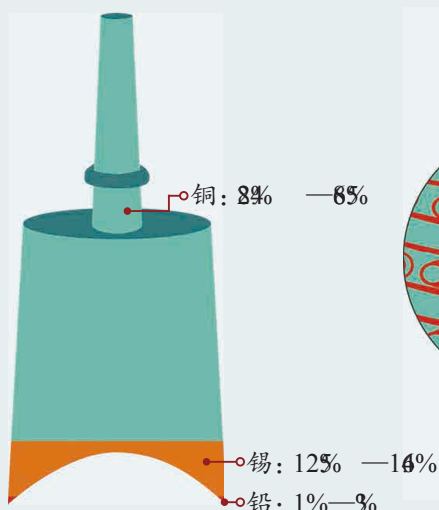
曾侯乙编钟成分
