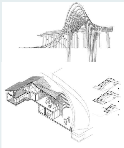
牛背山志愿者之家(设计图纸)
